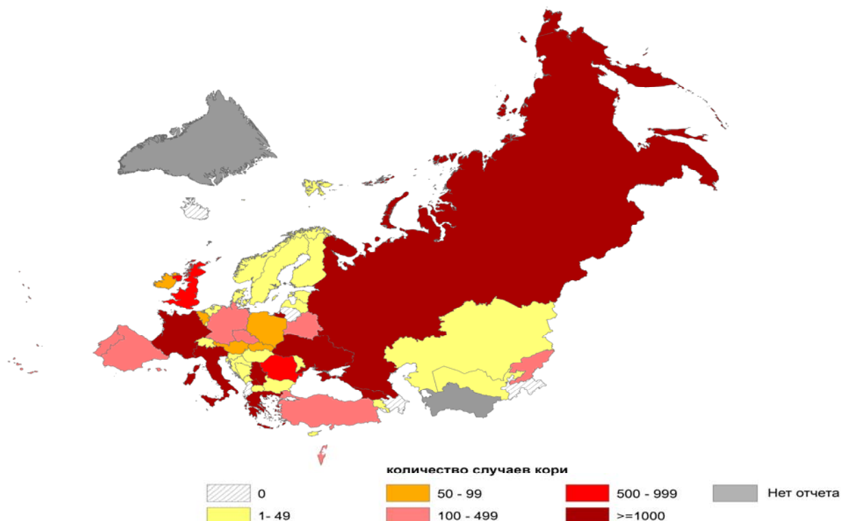
Рис. 1. Карта со случаями кори в Европейском регионе, Январь — Июнь 2018 г. (n=41013) (данные по состоянию на 01 Август 2018 г.)*
